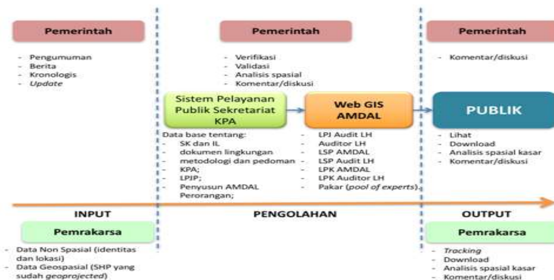
Bagan 7. Bisnis Proses Sistem Pelayanan Publik Sekretariat Komisi Penilai AMDAL dan Dokumen Lingkungan Hidup Lainnya
